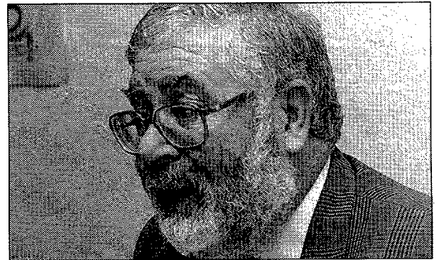
NOTICIAS
