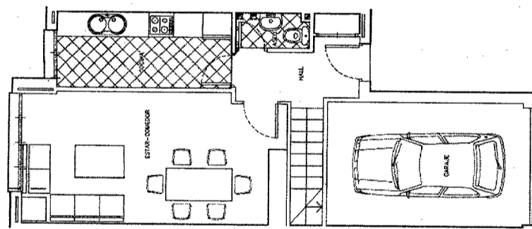
Planta Baja
