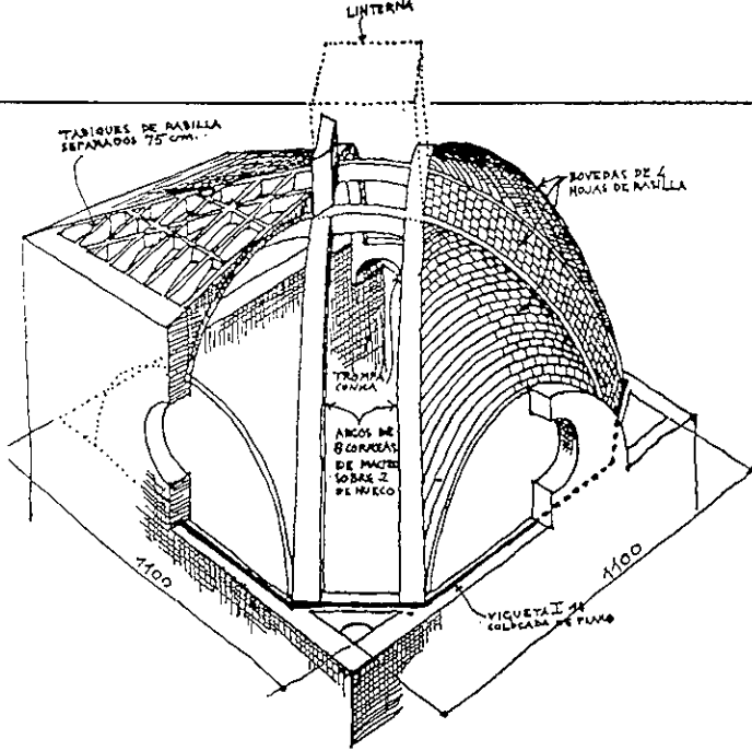
Iglesia de Manzanares. Cúpula de arcos cruzados de 13,30 metros de luz sobre caja cuadrada, con linterna
