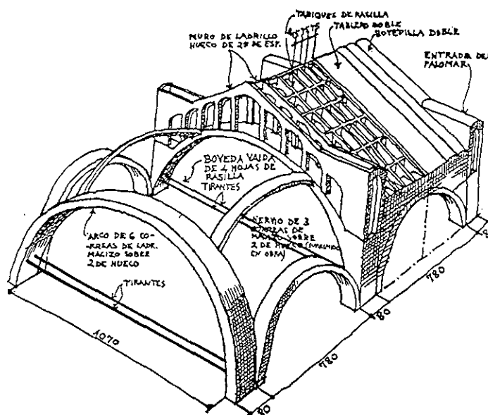
Nave compuesta de tramos de bóvedas vaídas, con los arcos fajones, atirantados, con hierros redondos a la vista, y sosteniendo un palomar
