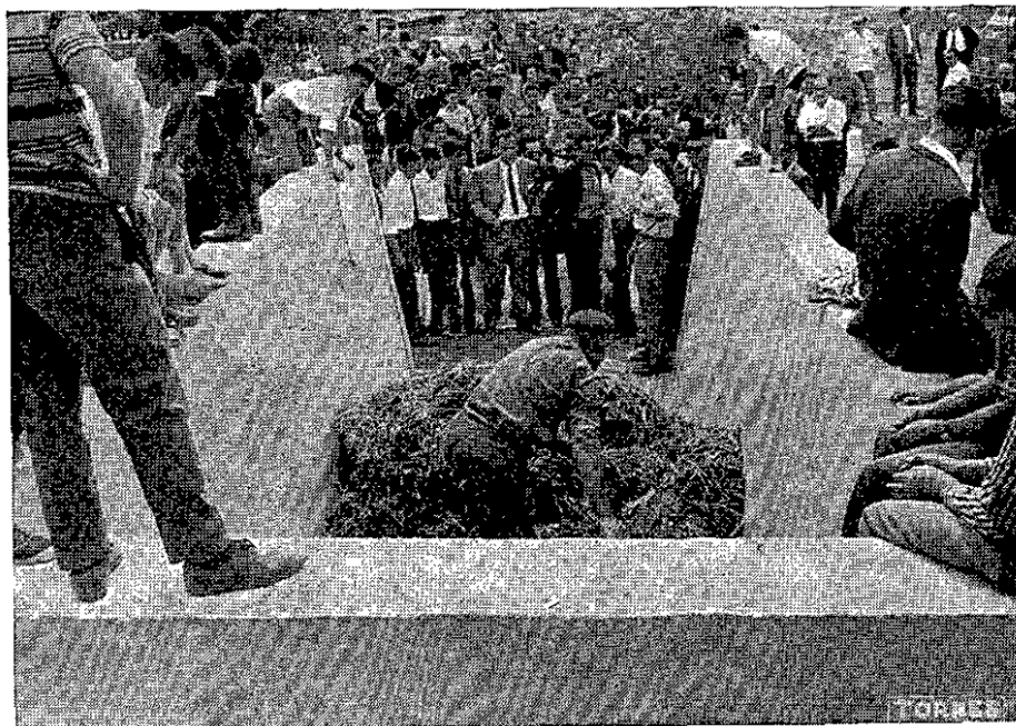
Ensilando el forraje en silo trinchera
