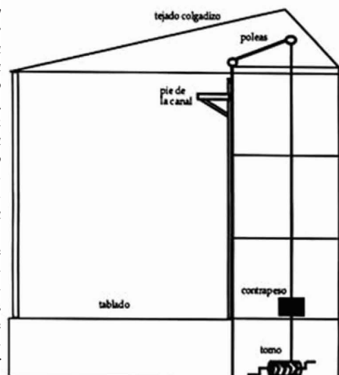
Hipótesis de funcionamiento de la canal en un corral de comedias. II. de José M a Ruano.
