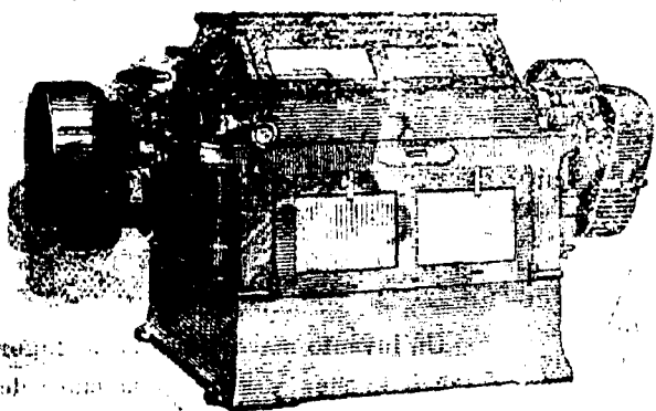
MOLINO MODELO D9 DE 4 CILINDROS OMAR PRIVILEGIO BUHLER
