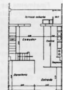
Planta baja de casa barata de dos pisos
