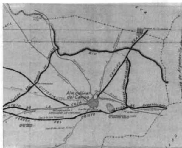
En trazo grueso pueden apreciarse algunas de las cañadas, cordels y veredas que se encuentran en los alrededores de Almodóvar del Campo
