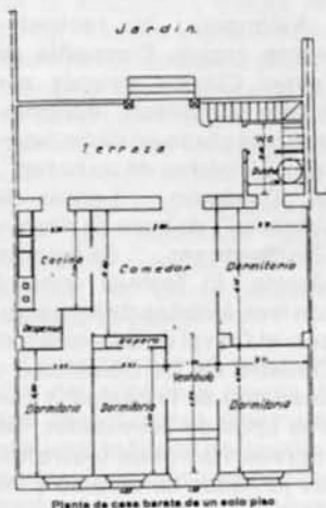
Planta de casa barata de un solo piso
