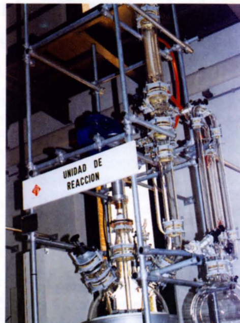
Instalación de planta piloto para la simulación del proceso industrial
