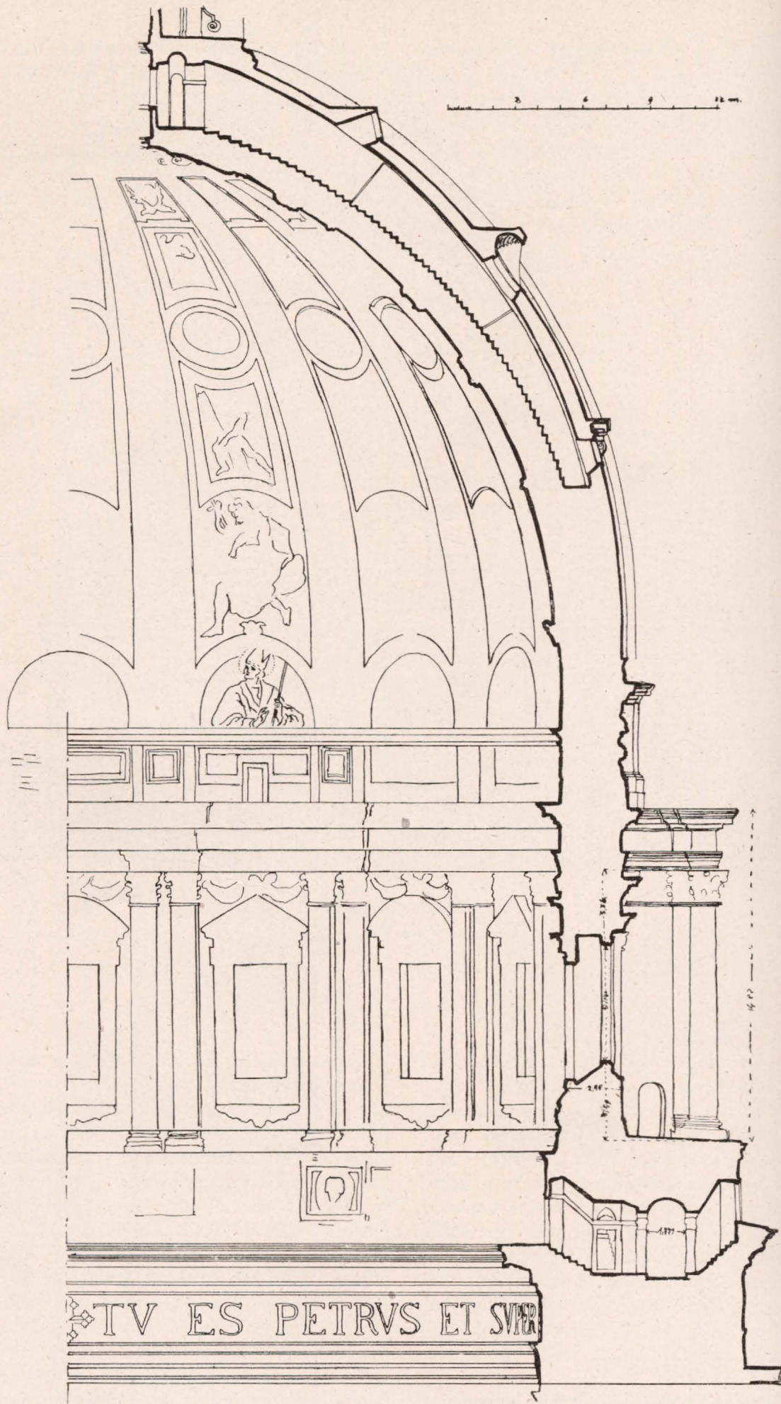
Sección de la gran cúpula.
