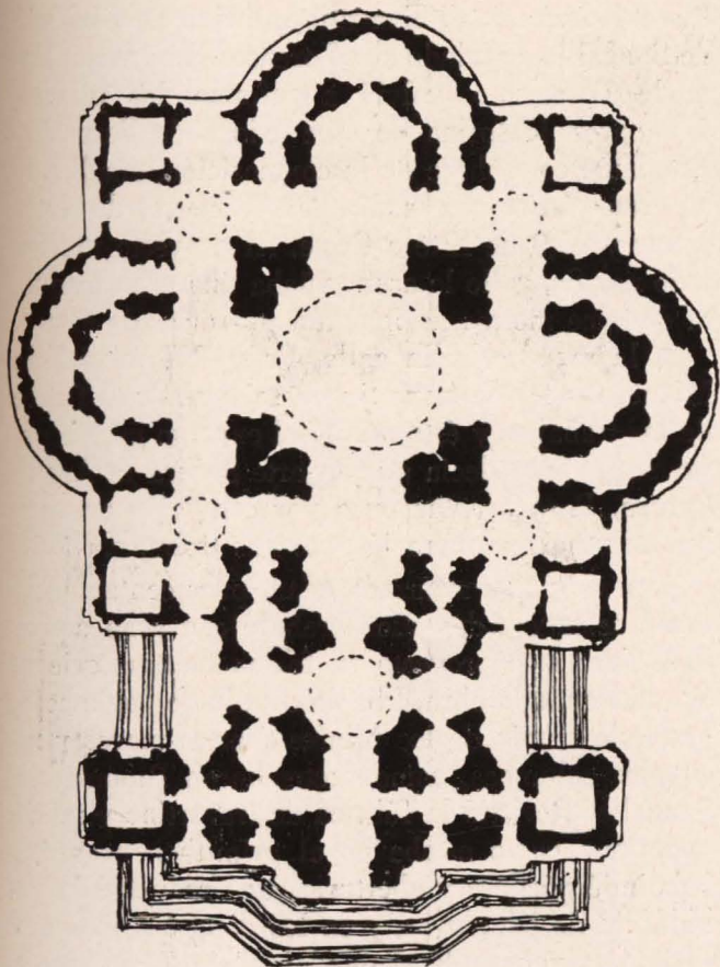
Proyecto de planta atribuido por Serlio a Rafael.
