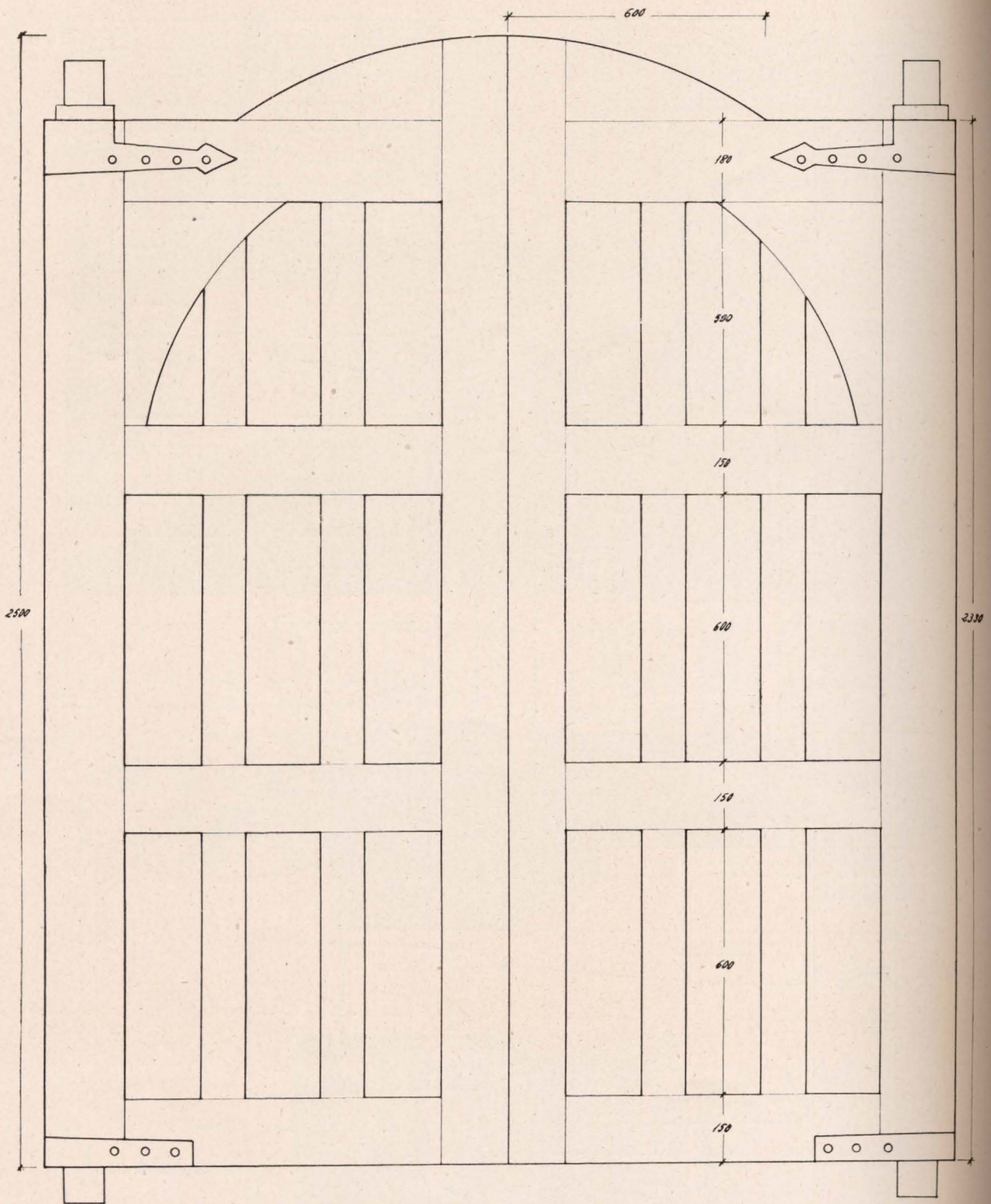
Puerta exterior. Leon. Astorga.
