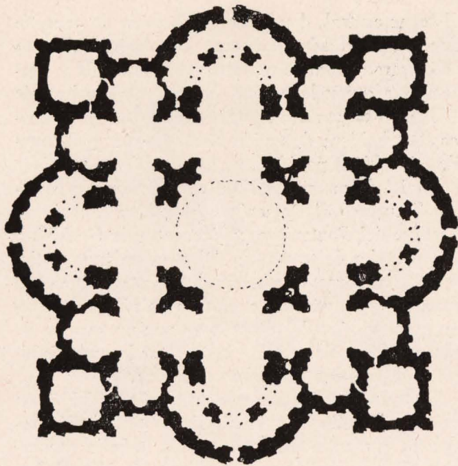
Proyecto de planta atribuida por Serlio a Peruzzi.
