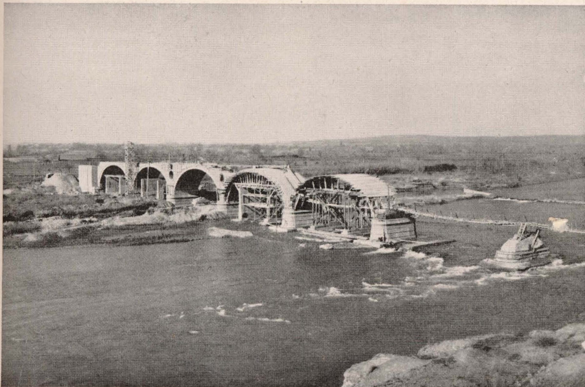
VILLANUEVA DE LA BARCA.—Puente sobre el río Segre y viviendas de nueva planta.
