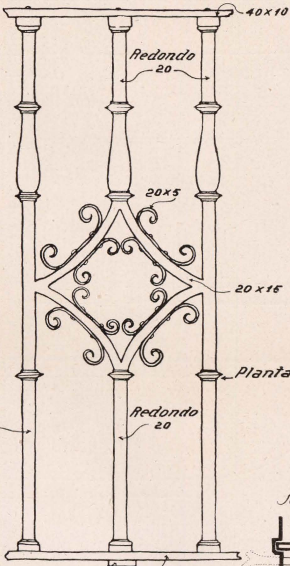
Balcón Leon. Astorga.
