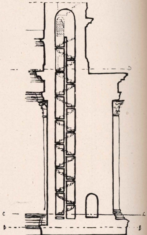
Sección del tambor por el pilar.
