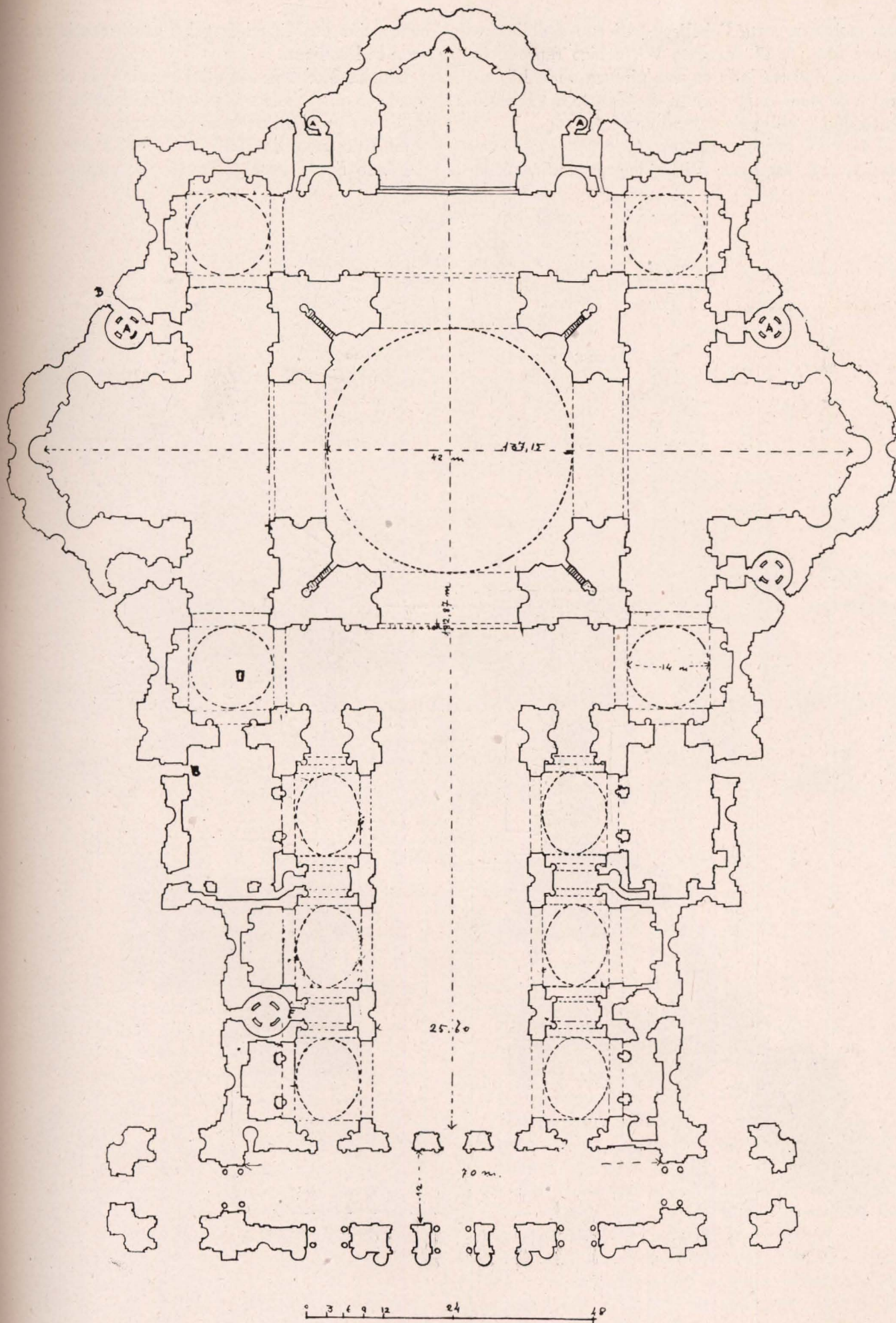
Planta actual de la Basilica de San Pedro.
