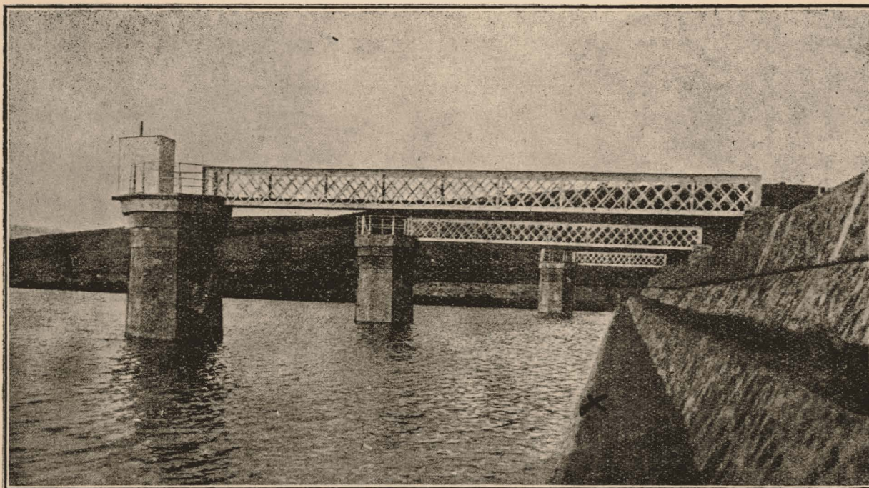
Puentes de servicio de las torres y escalonado de agua arriba de la presa. × La huella del escalón inferior, que está á la vista, enrasa con el umbral de los aliviaderos.
