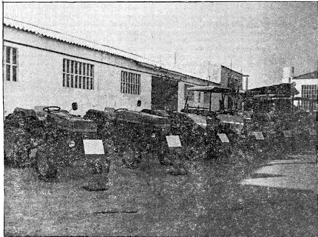
Exposición de los nuevos modelos de la serie 40 en el patio de las instalaciones de John Deere en Talavera
