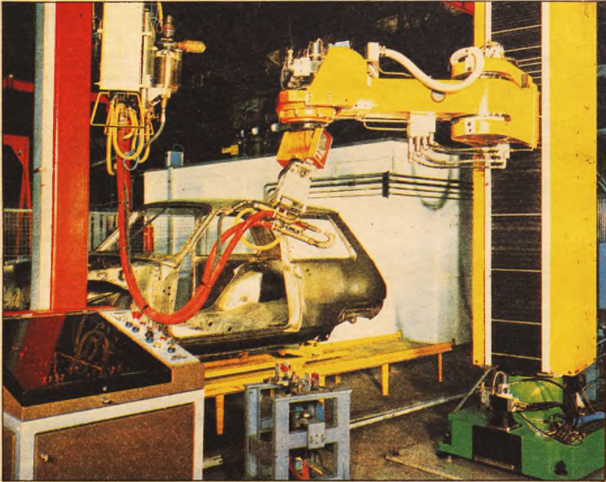
Un robot de soldadura, según seis ejes (coordenadas cilíndricas y ángulos de Euler), en funcionamiento en la Régie Nationale des Usines Renault
