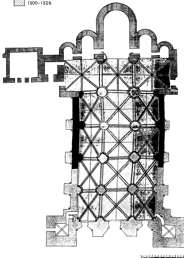
FIG. Nº XXII.- Planta de la catedral de Sigüenza, etapas constructivas desde la mitad del siglo XII a 1326. (María del Carmen Muñoz Parraga, La catedral de Sigüenza).
