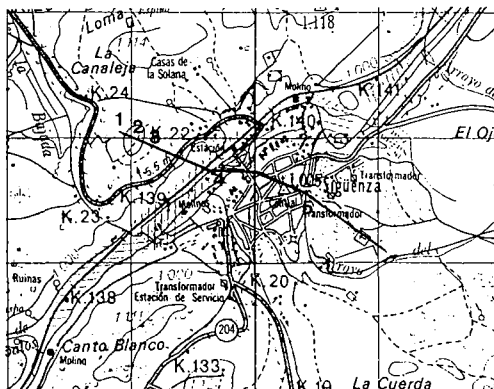
Fig. 4.- Perfil topográfico del transecto con localización de las muestras y dirección de los vientos locales.
