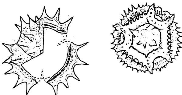
Fig. 2.- Esquema de granos de polen de compuestas.
