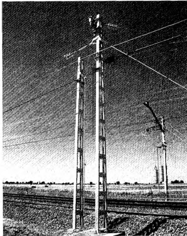
Obras del tramo Alcázar-Manzanares. En la foto se puede ver que las columnas de electrificación que había en el tramo Alcázar-Manzanares son iguales a las que se están instalando nuevas, además de colocarse en el mismo sitio. Se podría decir que casi estorban las viejas para instalar las nuevas. La columna que aparece al fondo es original y se cambiará cuando levanten esa vía. Las que se encuentran en primer término, la de la izquierda, es la vieja, y la de la derecha, la cambiada.
