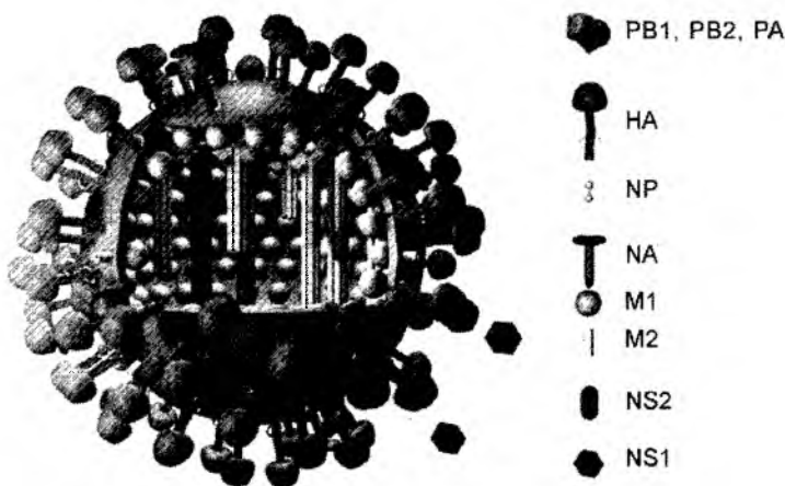
Esquema del virus H1N1.
