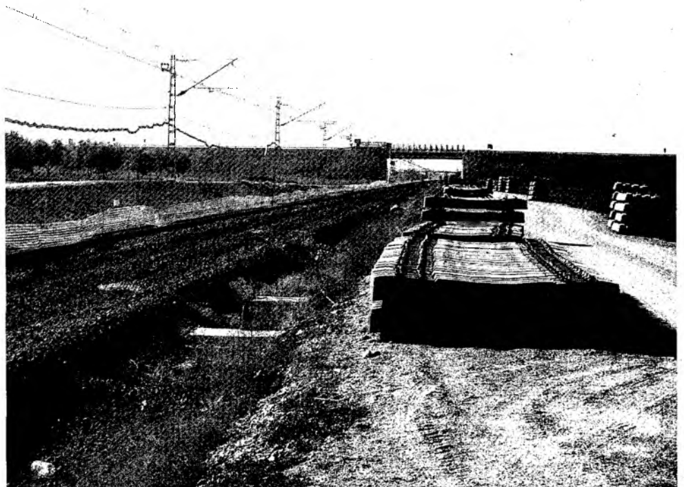
Obras del tramo Alcázar-Manzanares de la línea Madrid-Jaén.
