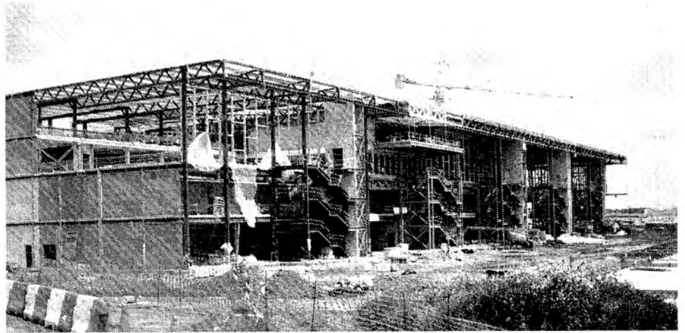
Obras de uno de los edificios del Aeropuerto de Ciudad Real.
