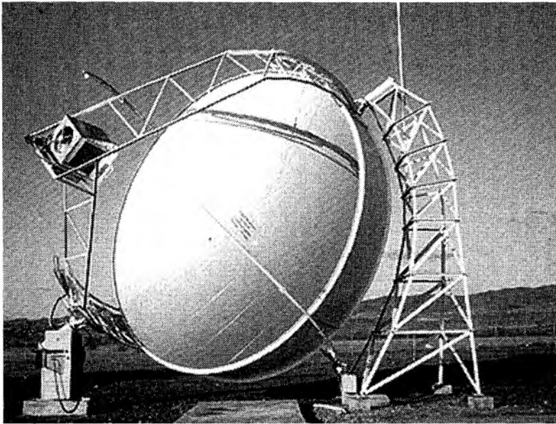
Sistema DISTAL I en operación en la Plataforma Solar de Almería.
