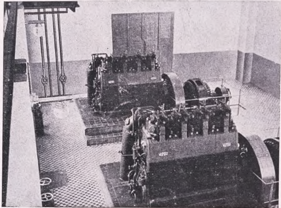
Pantano de Cijara (Extremadura). Central Termoeléctrica con alternadores tipo «Westinghouse» de 375 KVA cada uno
