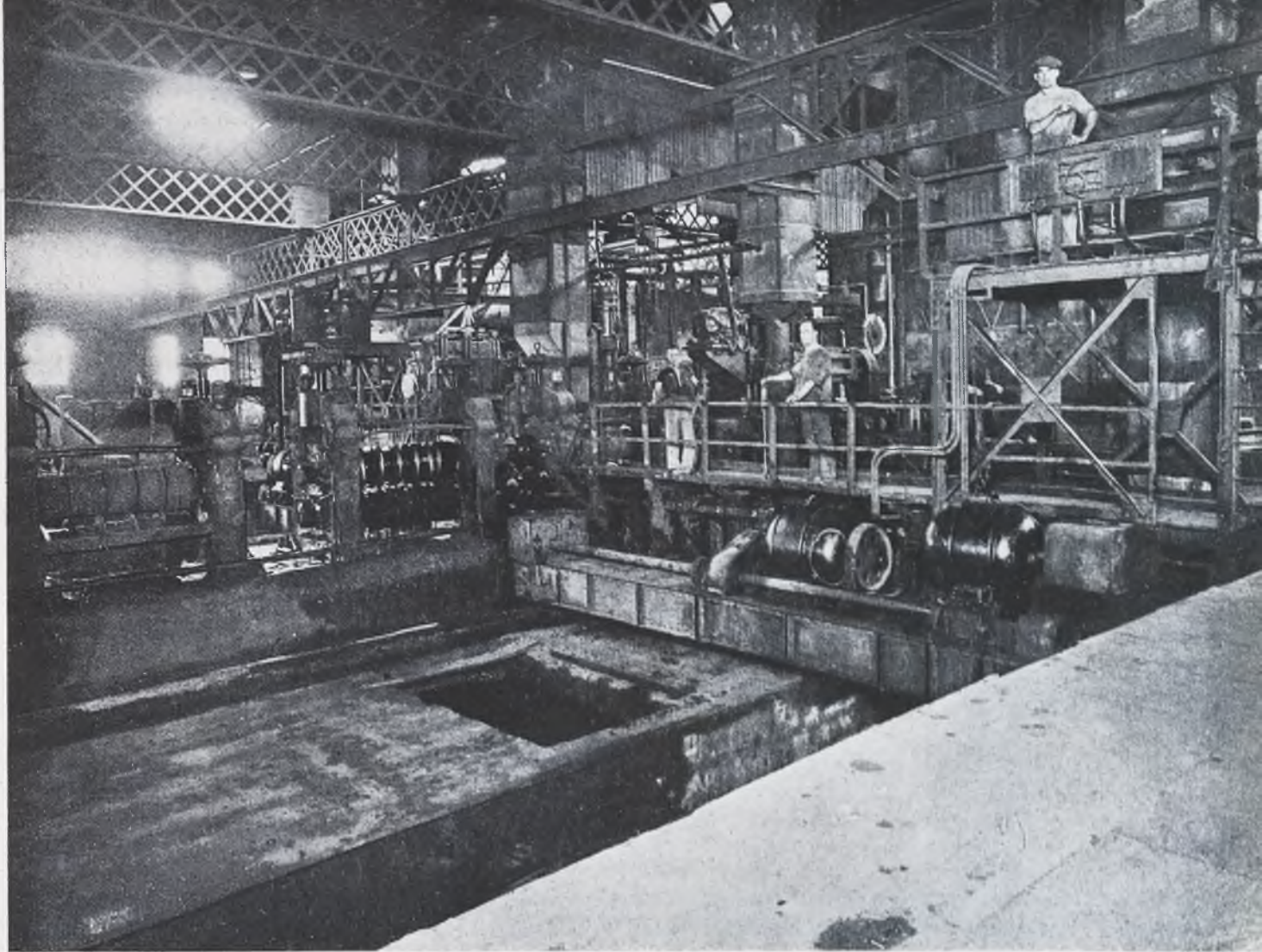
Laminación: tren de 650 mm. reversible y Blooming.
