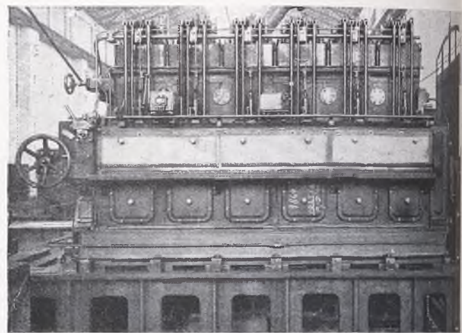
Un modelo de motor Diesel marino tipo Krupp, de 315 H. P., para pesqueros, que se construye en Barcelona.
