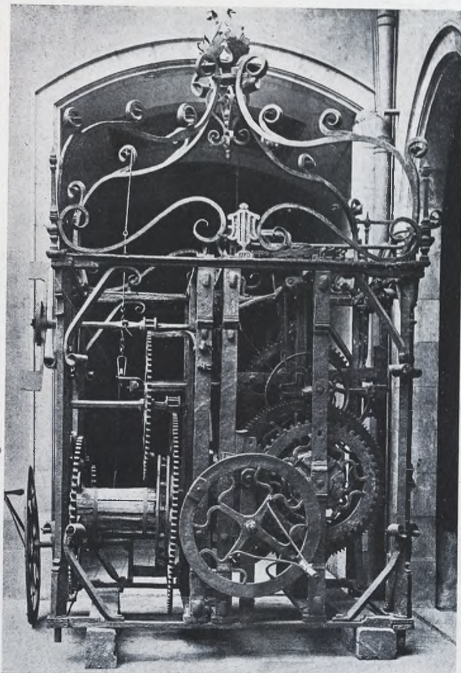
Alaquinería de reloj de fines del siglo XVI.
