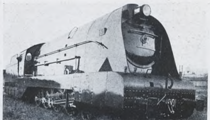
Locomotora tipo 1800 para los ferrocarriles M. Z. A., construida en Barcelona.
