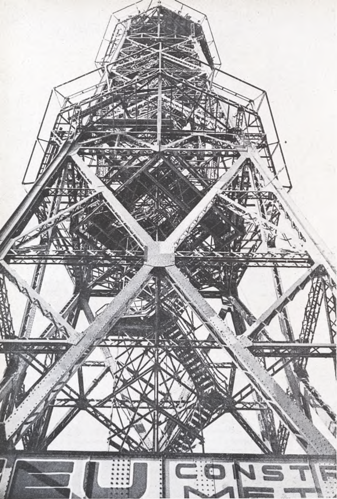
Torre de Jaime I del ferrocarril aéreo de San Sebastián a Miramar, construida en unos talleres de Barcelona.
