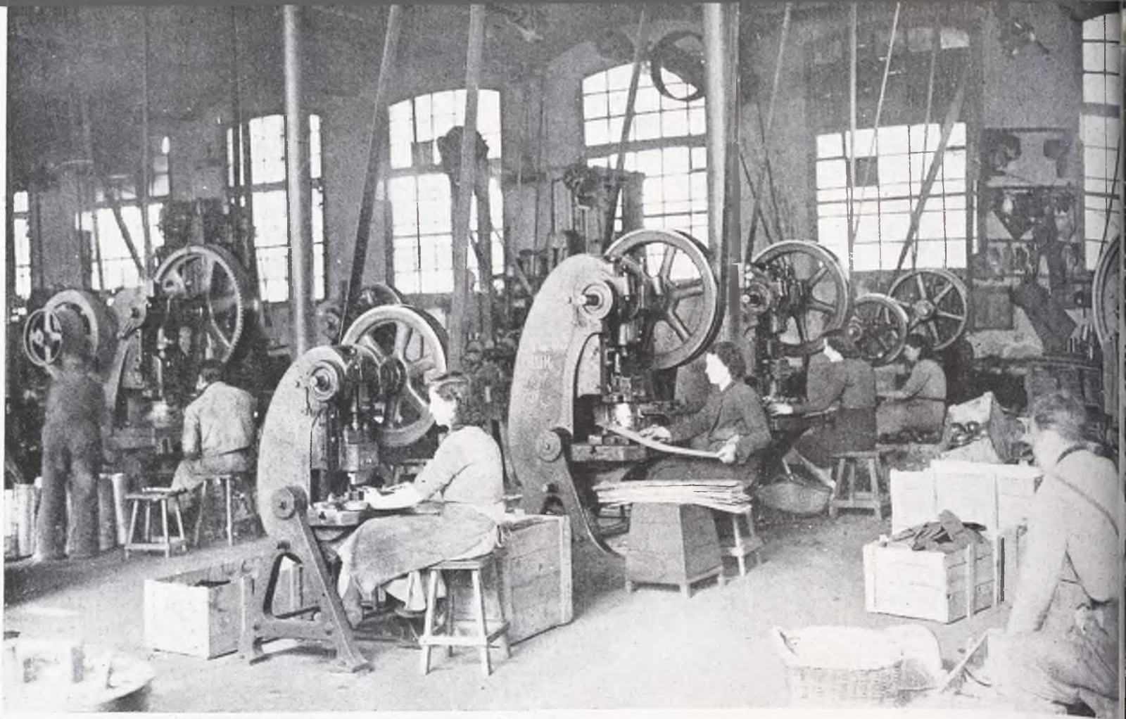
Sección de cortadoras en una fábrica de transformación de metales no féreos.
