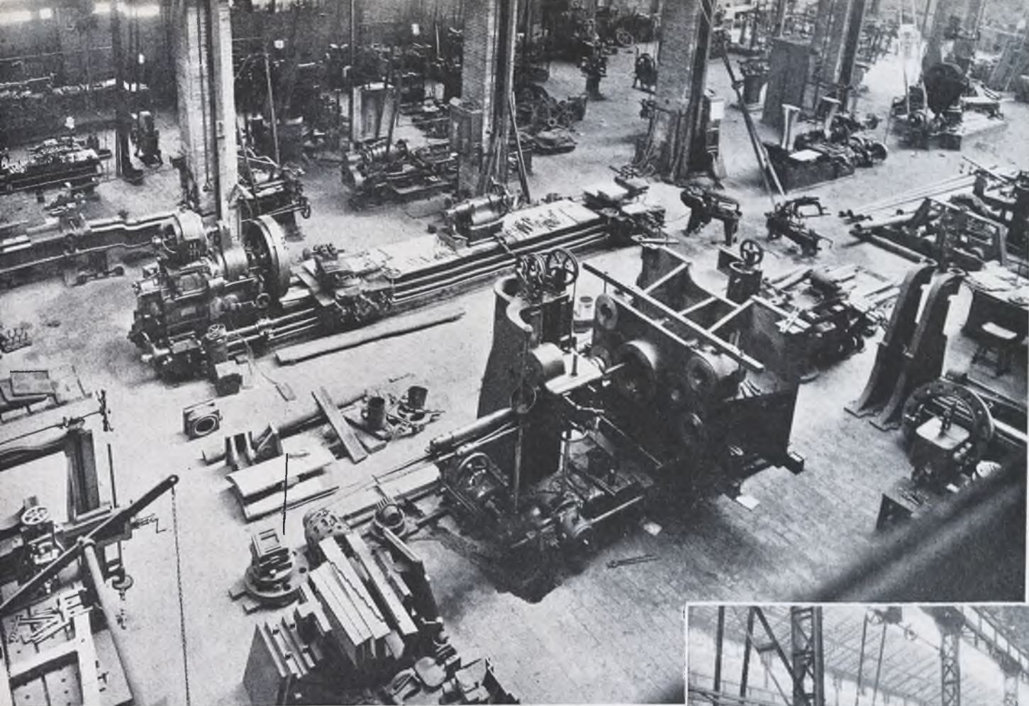
Nave de unos talleres especializados en la construcción de prensas y bombas hidráulicas para forjar, embutar, en diversas industrias.
