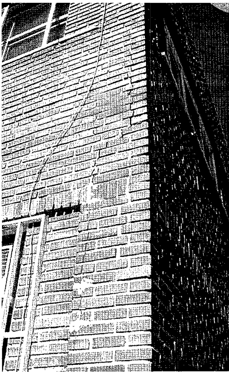
Esta grieta de apertura progresiva que aprecia en uno de los muros del edificio. En la imagen inferior de la derecha, agrietamiento del asfalto del aparcamiento de urgencias consecuencia del corrimiento de tierras.
