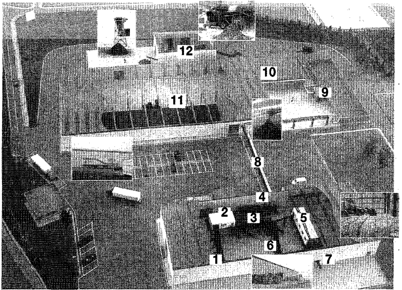
La maqueta reproduce fielmente la instalación, y sobre la misma, pequeñas fotos de los lugares indicados. Del 1 al 7 se refleja el proceso de selección de residuos, que llegan al nivel de empaquetado en los productos reciclables y contenerización del "rechazo"; del 8 al 12, el proceso de fermentación de residuos orgánicos, y posterior depuración del compost resultante, así como depuración del aire.
