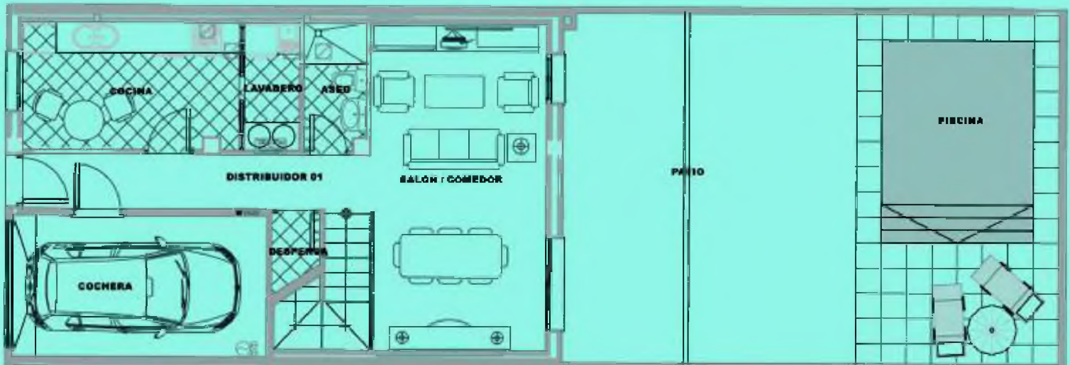
PLANTA BAJA
