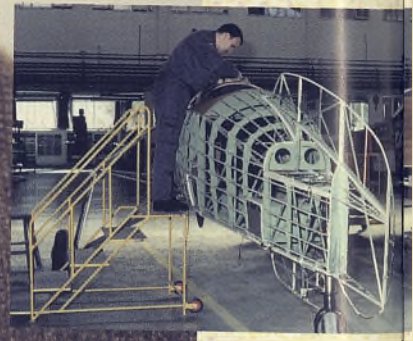
En plena construcción del C-30 en la Maestranza
