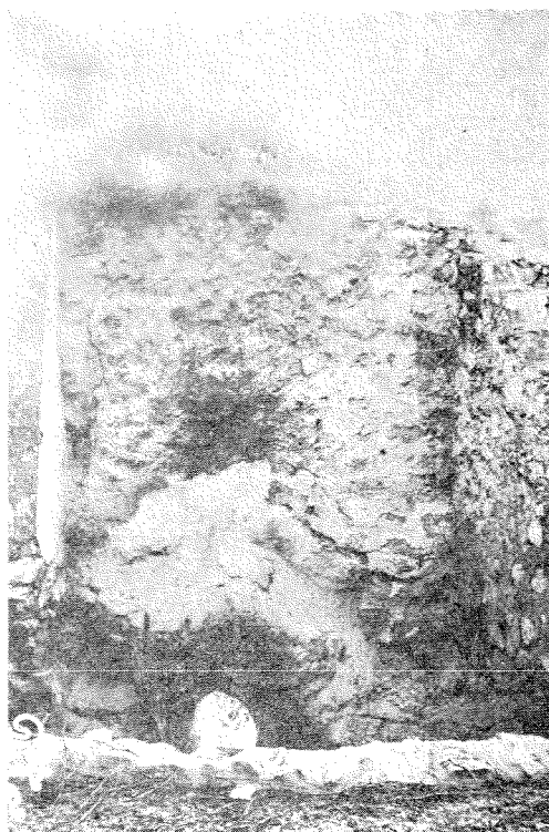
El barranco y la boca del horno. El medio punto de la parte inferior es la boca y la claridad que se aprecia en su fondo es debida a las llamaradas de las gavillas que arden.
