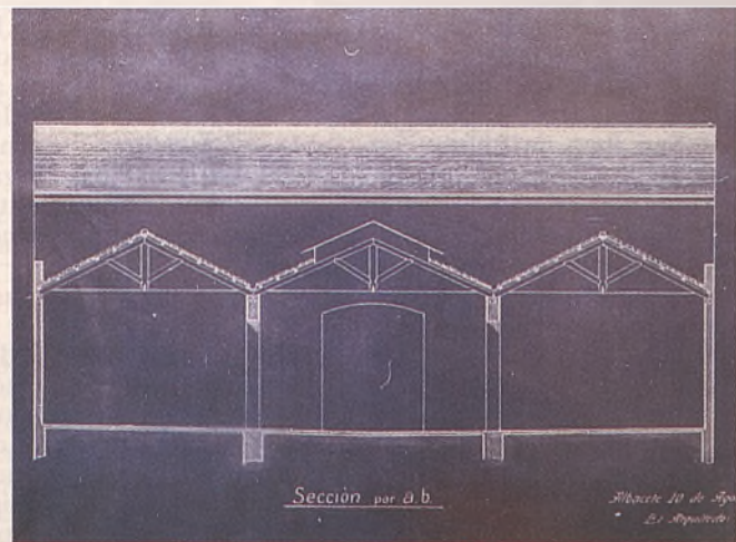
De izquierda a derecha, alzado y sección del garaje proyectado por Julio Carrilero (1924) en el Barrio de la Industria.
