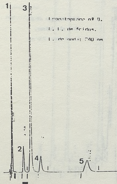
Cromatograma nº 7.
