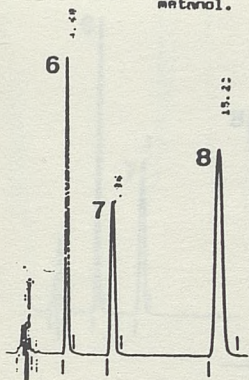
Cromatograma nº 5.
