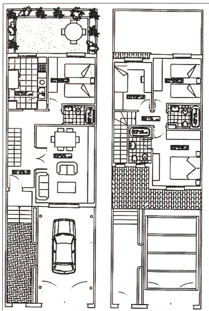
Planta baja
