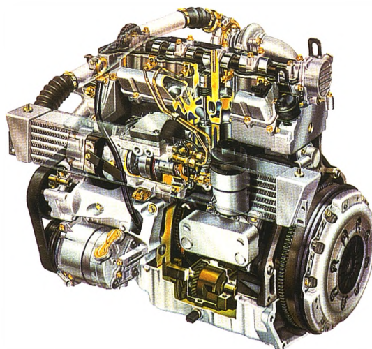
El motor transversal incorpora un intercooler para el aire de admisión, el cual asegura mayor potencia.
