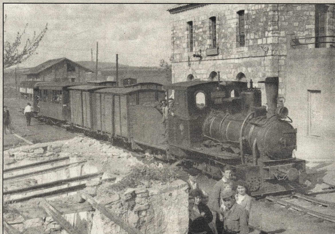
Locomotora n.º 6 (Asturias), con un tren mixto en la estación de Calzada. «Vía estrecha en España». MAF
