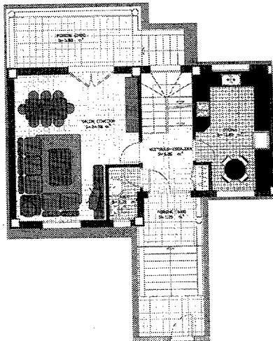
PLANTA BAJA
