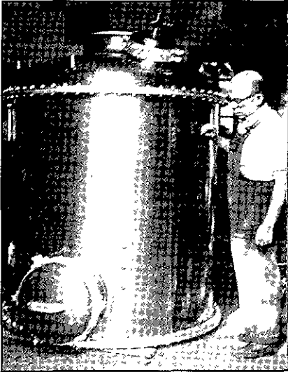
Caldera alambique, encargo de «Anís de la Asturiana» (1968) con Andrés, uno de los hijos del fundador
