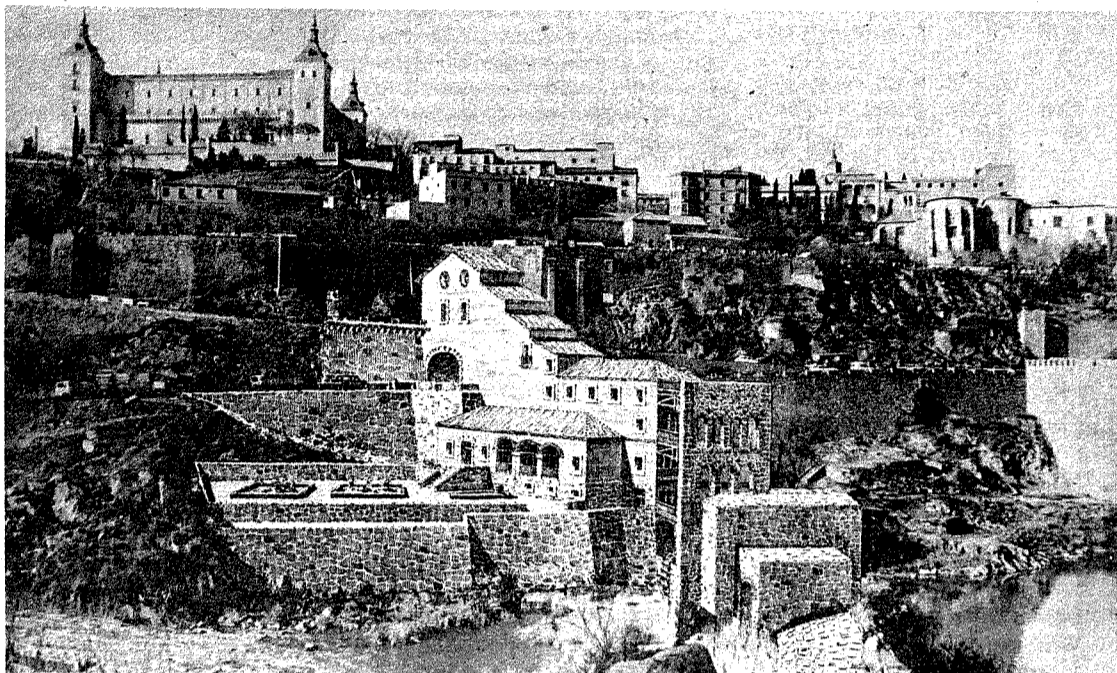
Aspecto general del proyecto de Juanelo Turriano de subida de agua desde el Tajo hasta la ciudad de Toledo. El proyecto data del siglo XVI.
