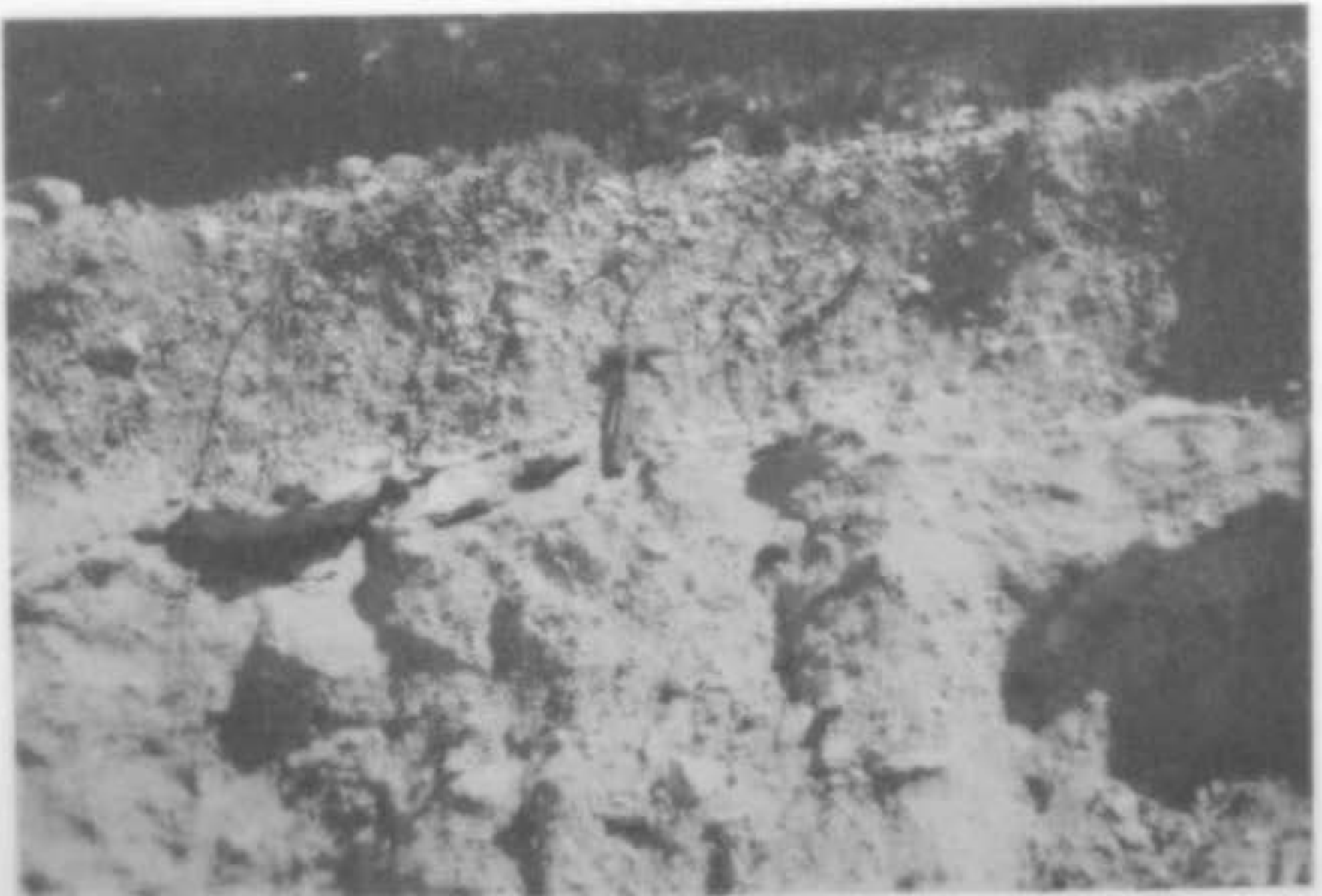
Foto 9: Suelo con costra calcárea. 3.ª Parada.
