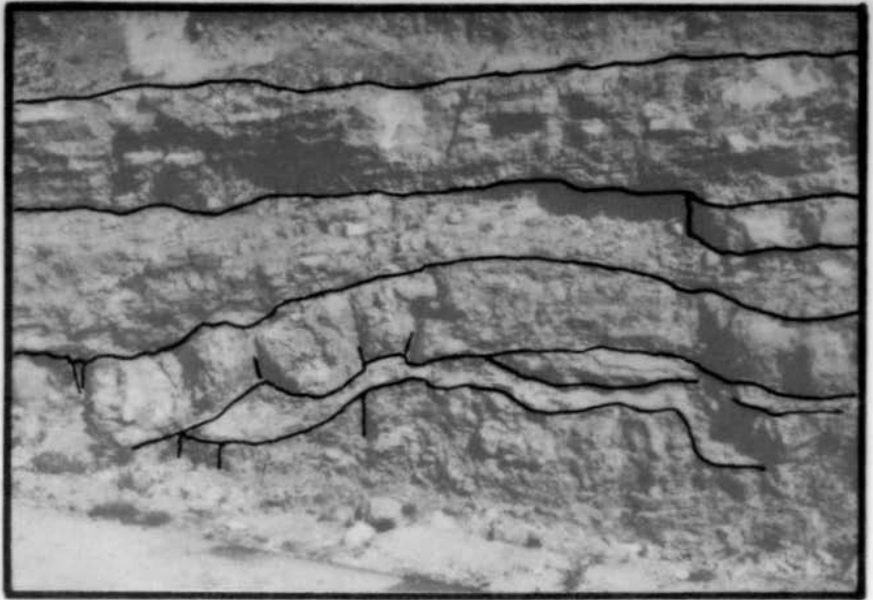
Foto 6: Repliegues en los materiales de la 3.ª Parada.
