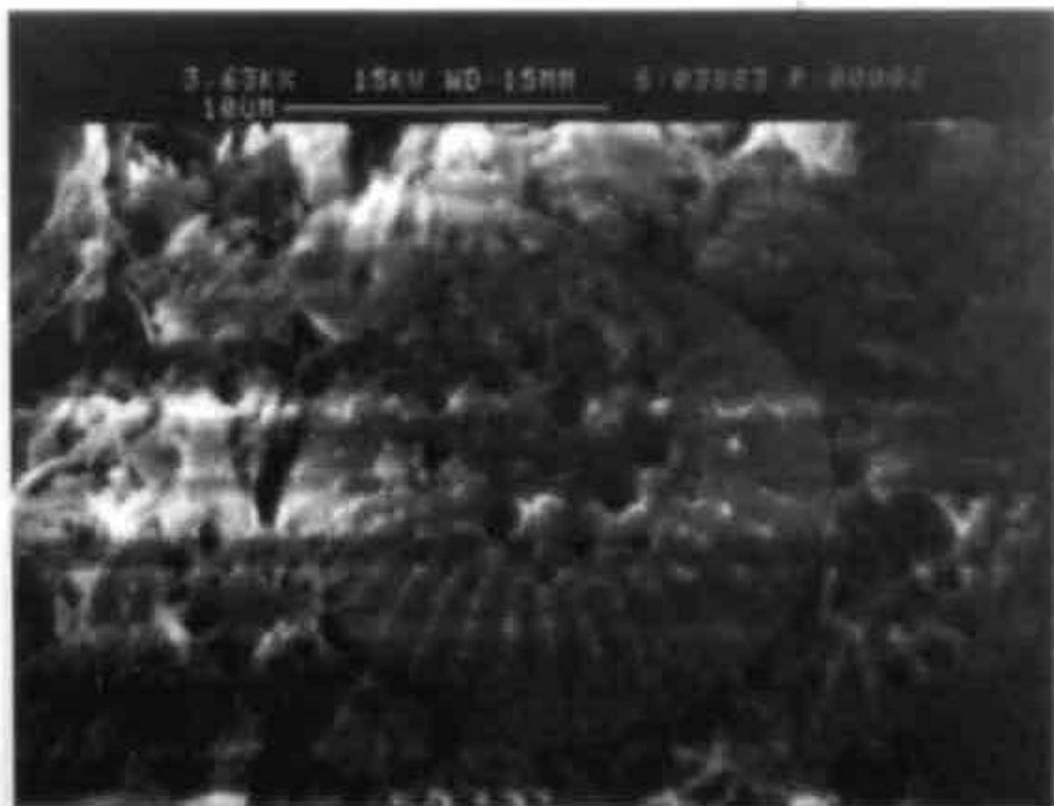
Fig. 43. Detalle de la figura anterior, en la que se observa una frústula de diatomea sin bien conservada. Imagen de Microscopía Electrónica de Barrido.
