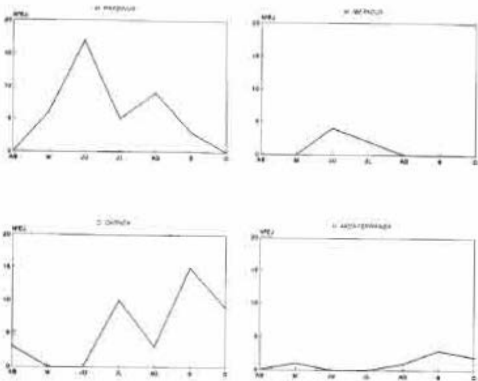
Fig. 15: Fenología de las cuatro especies más abundantes de la familia Chrysopidae en el conjunto de los biotopos estudiados.
