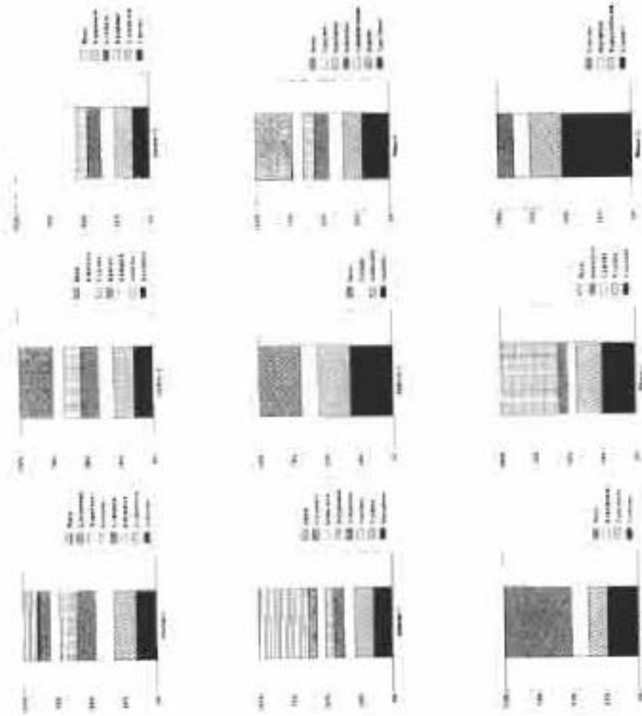
Fig. 4. Gráfico de barras representativo del porcentaje (en base a las óximizadas) con el que las especies más representativas contribuyen a la estructura de 40 comunidades (medios arbóreo o arbustivo).
