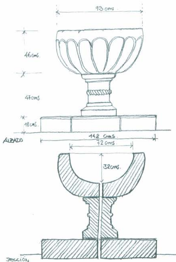
Fig. 3. Alzado, sección y medidas de la pila bautismal. (Antonio Peiró).
