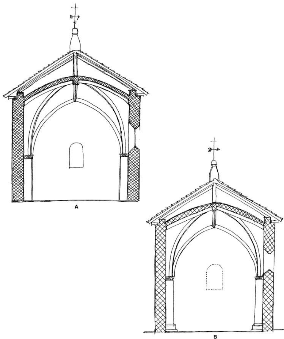
Fig. 4. Dibujos a mano alzada que muestran el nivel del presbiterio antes de la restauración (A) y después de la misma (B). (Antonio Peiró Amo).
