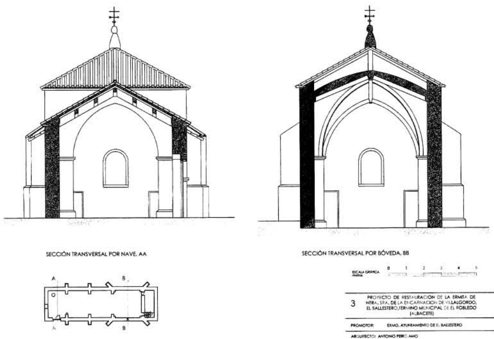
Fig. 1. Ermita. Secciones transversales.
