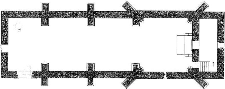
PLANTA GENERAL
