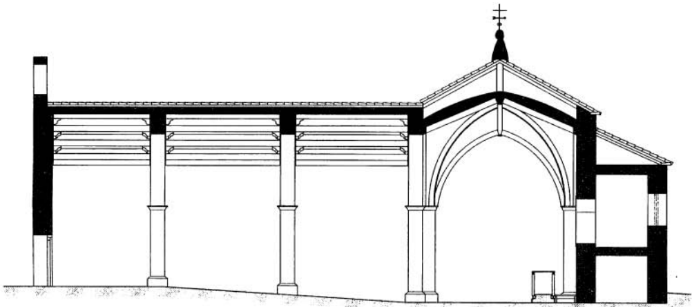
SECCIÓN LONGITUDINAL
