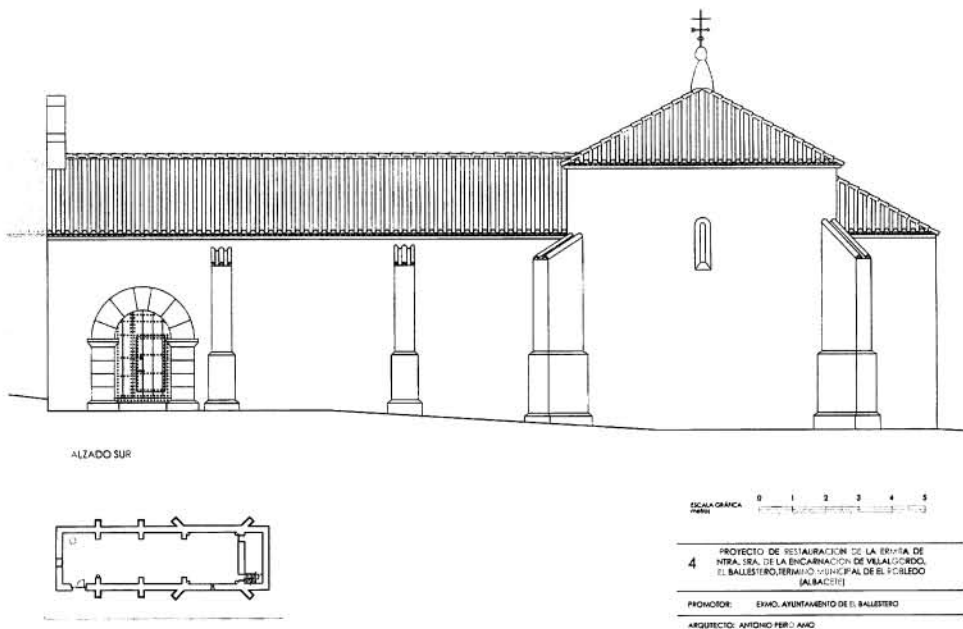
Fig. 2. Ermita. Alzado sur.
