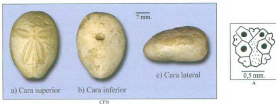
Figura 31. Eupatagus acuminatus , CFN. A. Sistema apical-plumilla.
