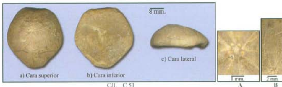
Figura 23. Pygurus jurensis , CJL. C 51 A. Sistema apical; B. Ambulacro III.
