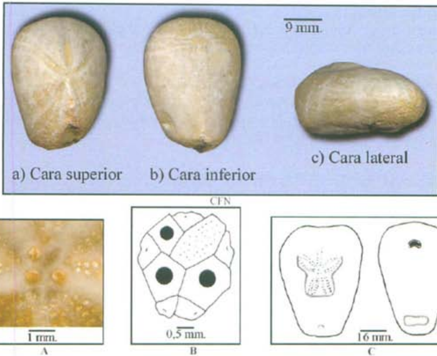
Figura 27. Cyclaster heberti CFN. A. Sistema apical; B. Sistema apical-plumilla; C. Fasciolas peripetalifera y subanal-plumilla.
