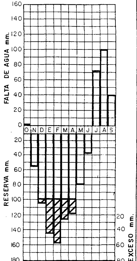
HISTOGRAMA DEL BALANCE DE HUMEDAD
