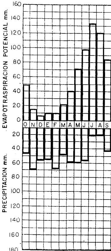
HISTOGRAMA DEL BALANCE DE HUMEDAD
