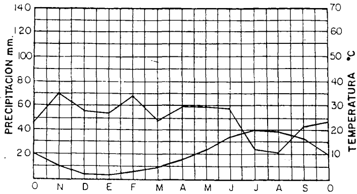
DIAGRAMA OMBROTERMICO (GAUSEN)
