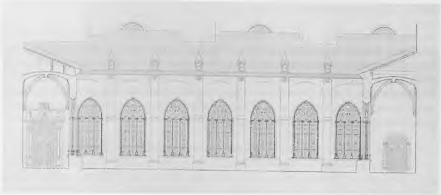
Fig. 13.- Claustro del siglo XVI: Planos de plantas, y alzado sur, con la restitución hipotética de su coronación original (del proyecto de restauración redactado por Eduardo Barceló y José Juste, y de la tesis doctoral del último) .
