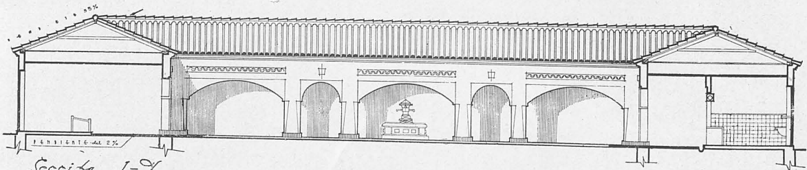
Sección I-II
