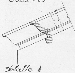
Detalle de la portada Escala 1:20
