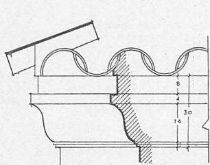
Detalle de la cornisa
