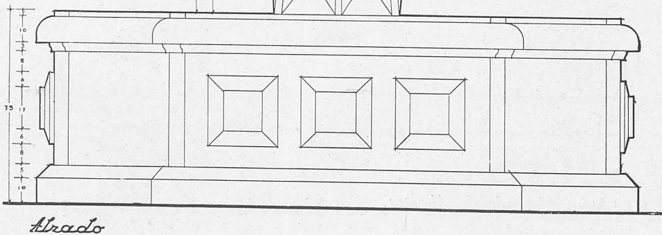
Detalle de la fuente Escala 1:40
