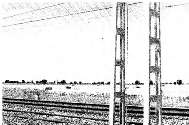
Obras de la línea en el tramo Alcázar-Manzanares.
