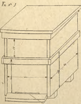
Figura 1. — Colmena con un alza. Consta de cuatro piezas acopladas por superposición: tablero, cuerpo de colmena o nido de cría, alza y tapa.
