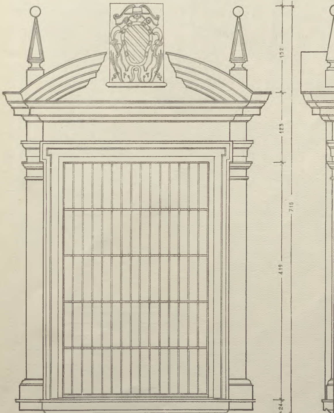
ALZADO
