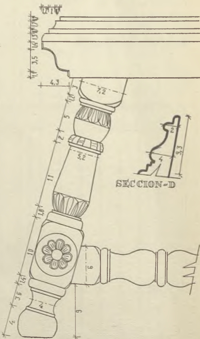
DETALLE. B~C
