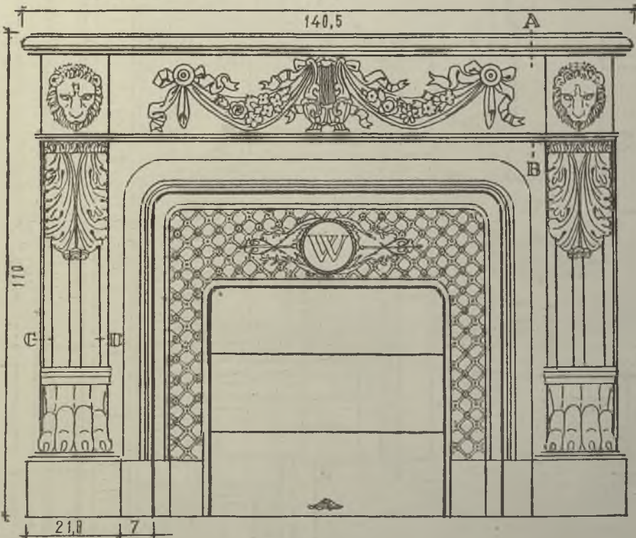
ALZADO
