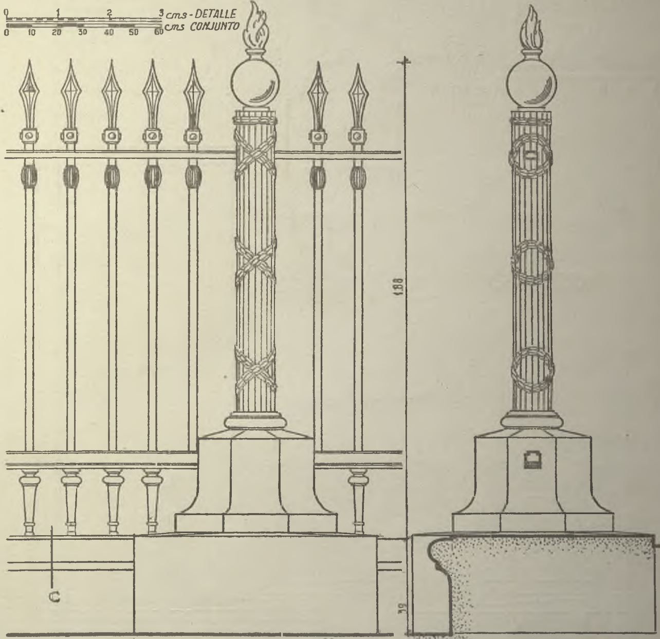
SECCION
