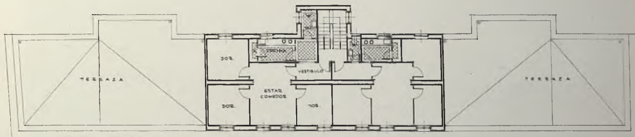
Planta de áticos
