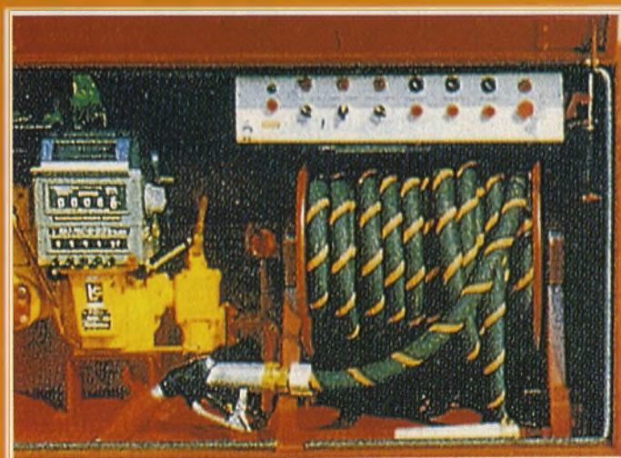
Detalle del contador homologado y mangueras de servicio.
