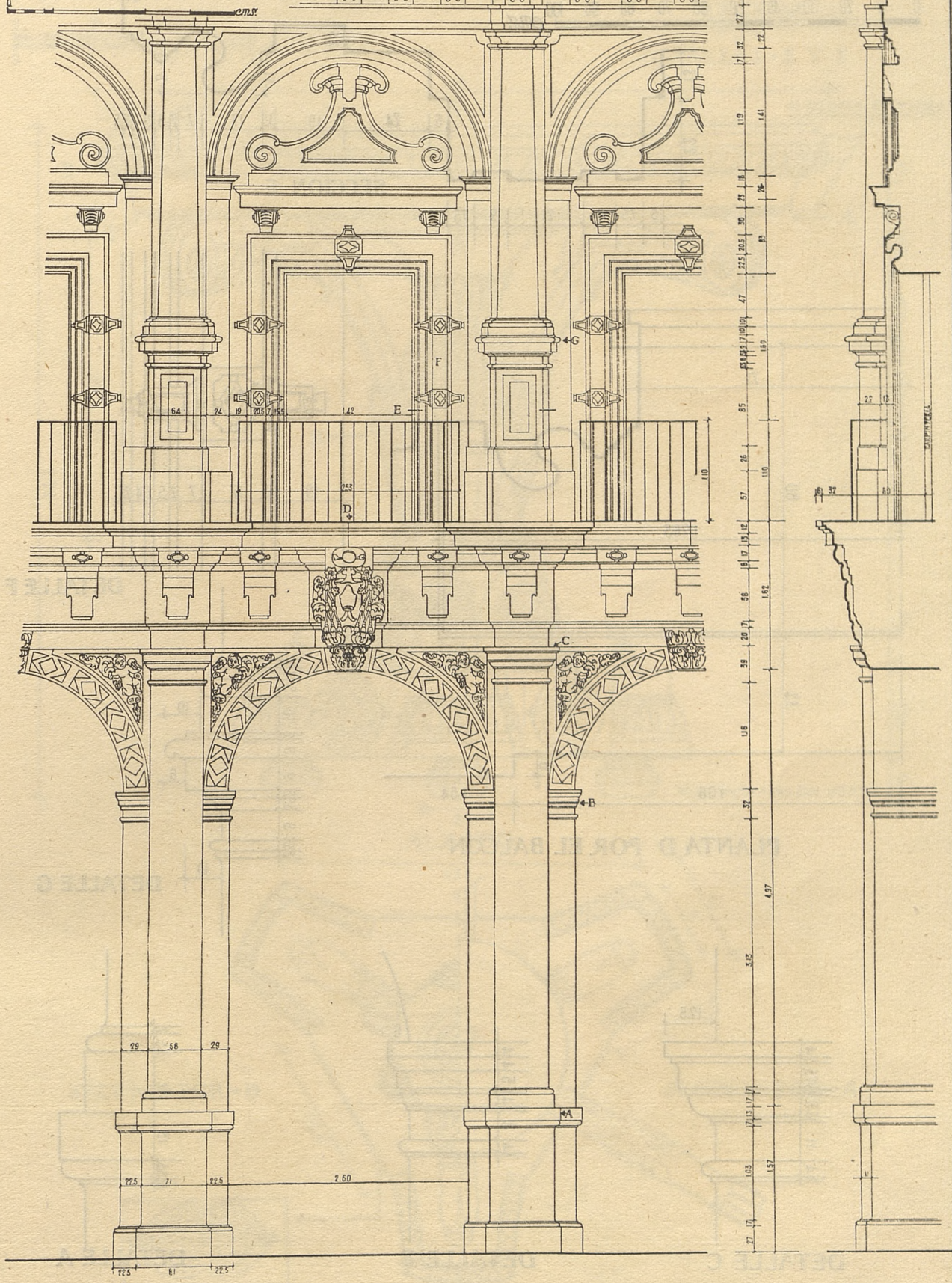
ALZADO FRONTAL
