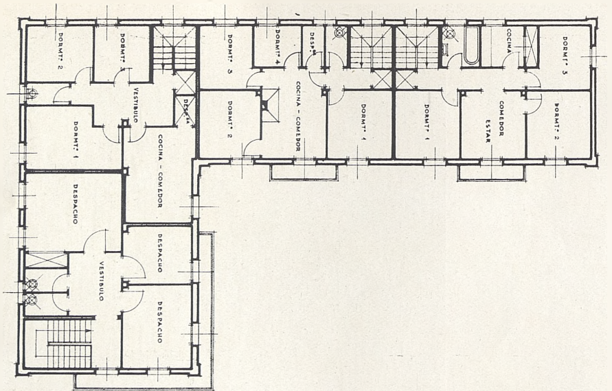
Planta principal
