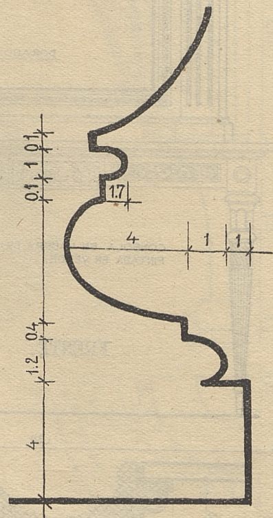
SECCION C-D
