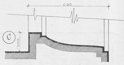
JAMBA. ESCALA 1:10.
