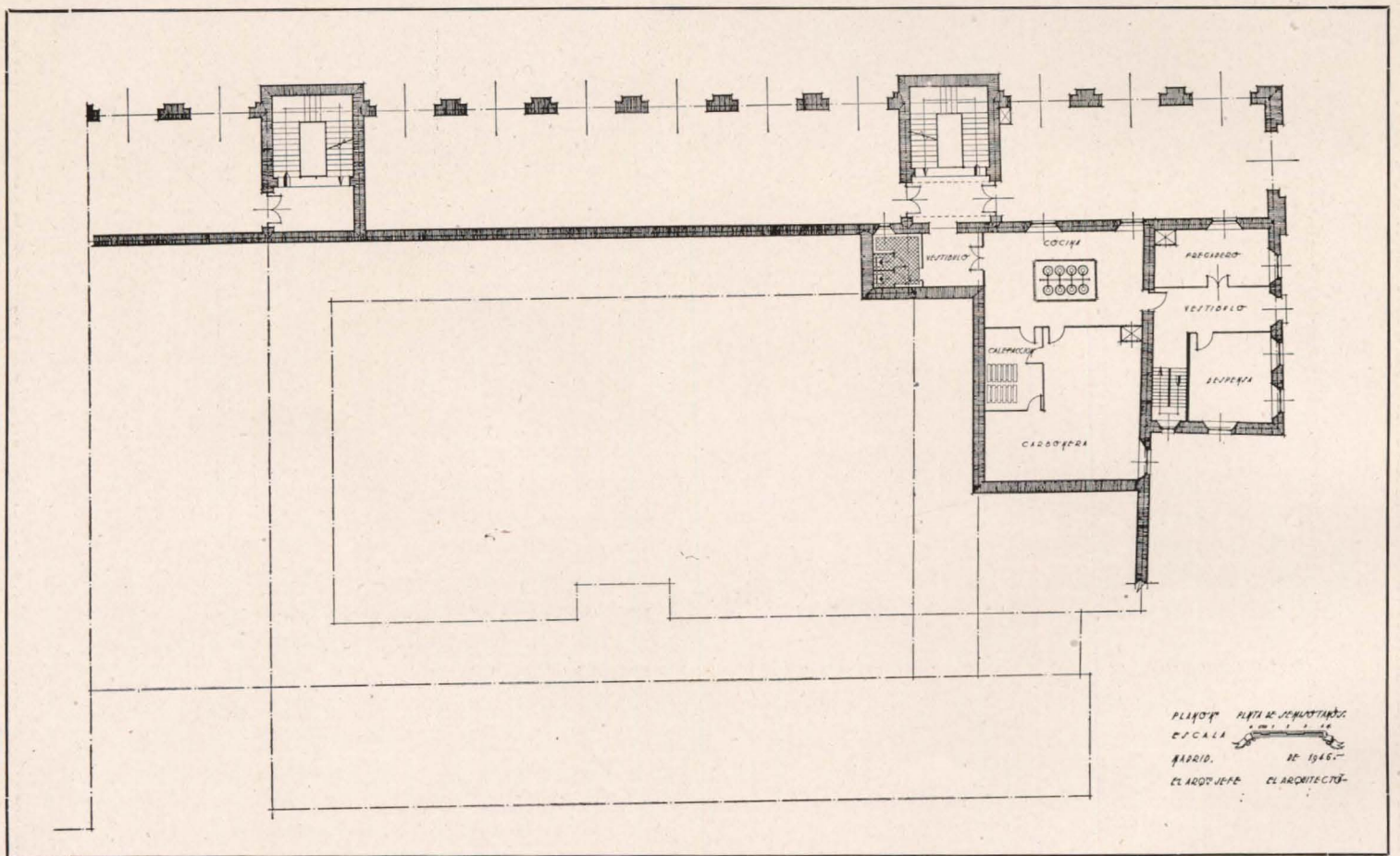
Planta baja y planta de semisótanos.
