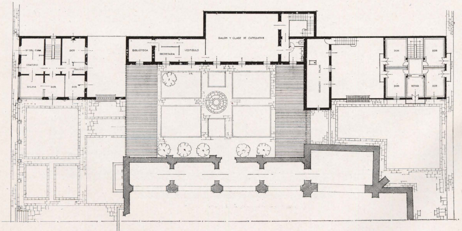
Anejos de la Iglesia. Archivo parroquial y vivienda y casa de labrador tipo 4-D. Alzado y plantas.
