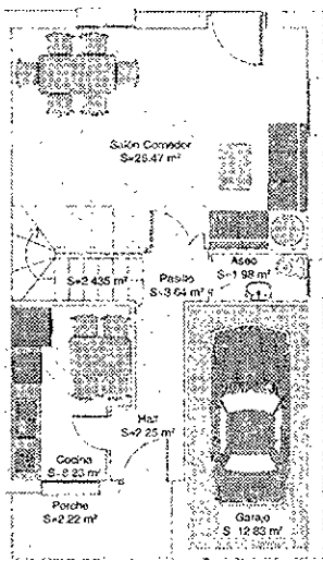
PLANTA BAJA Superficie Útil: 60.055 m 2 .
