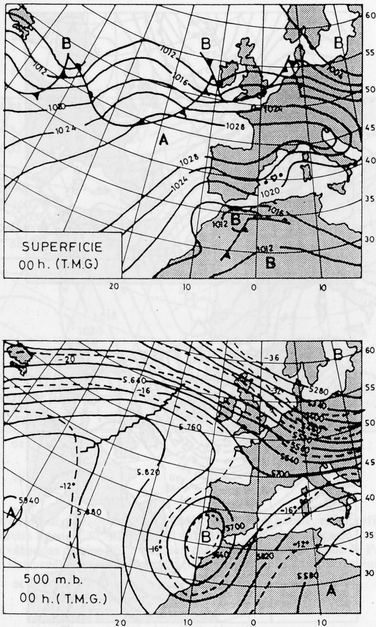
Fig. 4. Situación ciclónica de Levante en superficie y gota fría en altura (19-X-1973). Flujo de Levante (Este) en superficie sobre la Meseta y gota de aire frío sobre la vertical del cuadrante suroccidental de la Península. La presencia de esta perturbación en altura da lugar en ocasiones, como en el caso presente, a una ciclogénesis en superficie con irrupción en la Meseta de vientos húmedos de Levante. Es una situación atmosférica típica de lluvias intensas en la Meseta.
